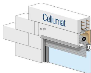
Gesloten rolluikkasten
